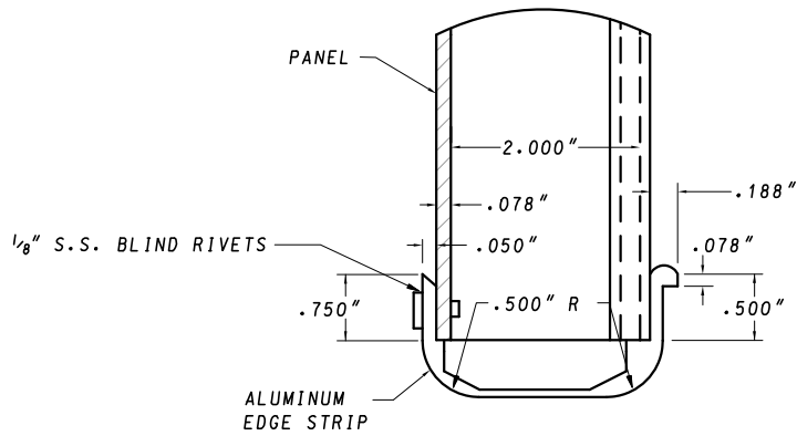
DETAIL OF EDGE STRIP
