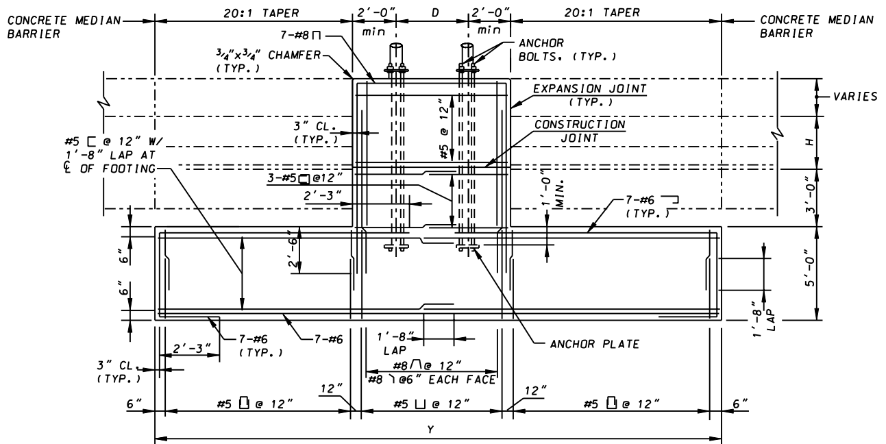
SECTION D-D
