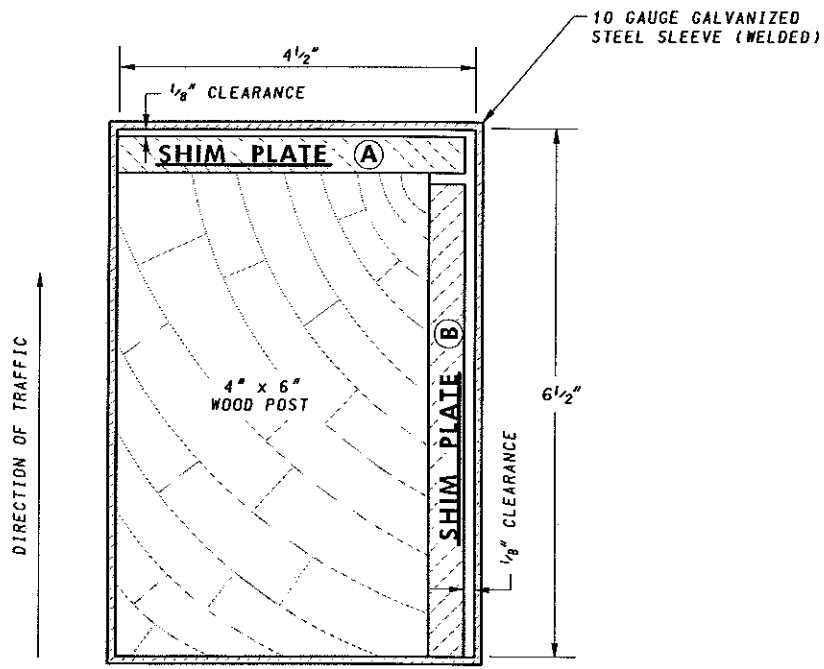
SECTION A-A
