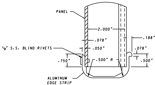
DETAIL OF EDGE STRIP
